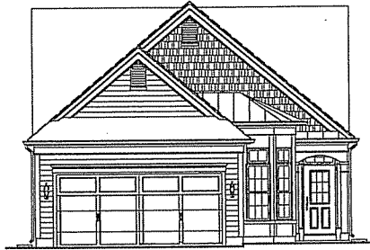
Elevation 60
