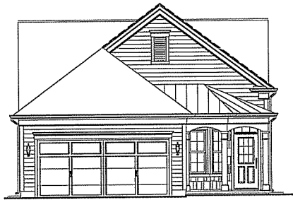
Elevation 1
