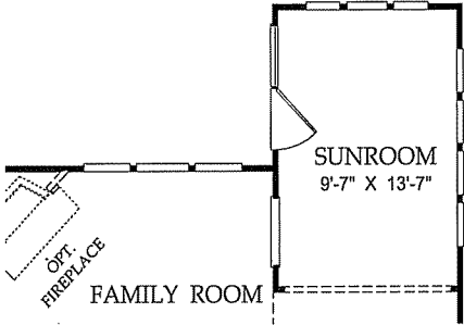
Optional Sunroom
